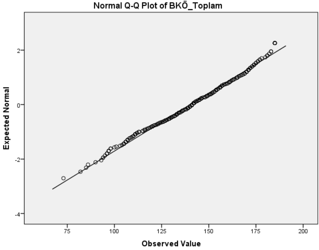
Şekil 6. Baba Katılım Ölçeği Q-Q Plot Dağılımı
