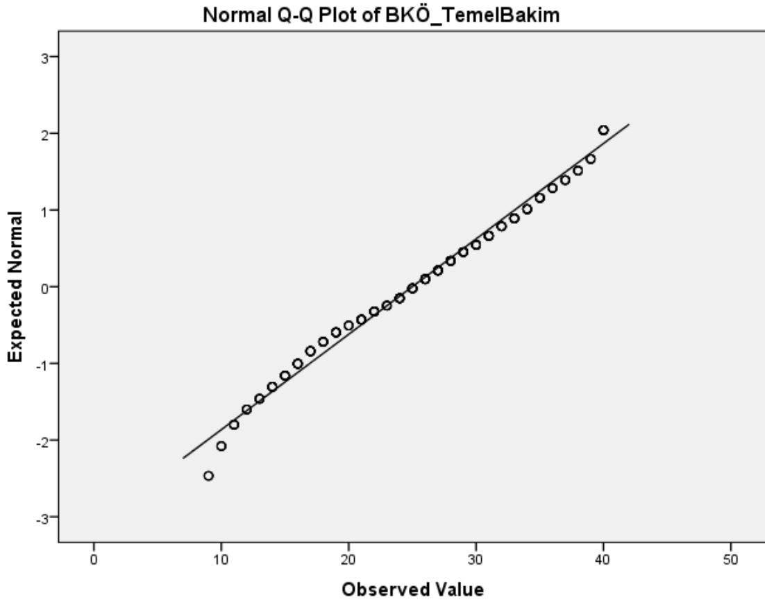
Şekil 9. Baba Katılım Ölçeği Temel Bakım Alt Boyutu Q-Q Plot Dağılımı
